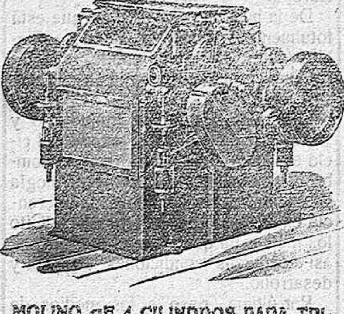
MOLINO DE 4 CILINDROS PARA TRIATURACIÓN O COMPRESIÓN
