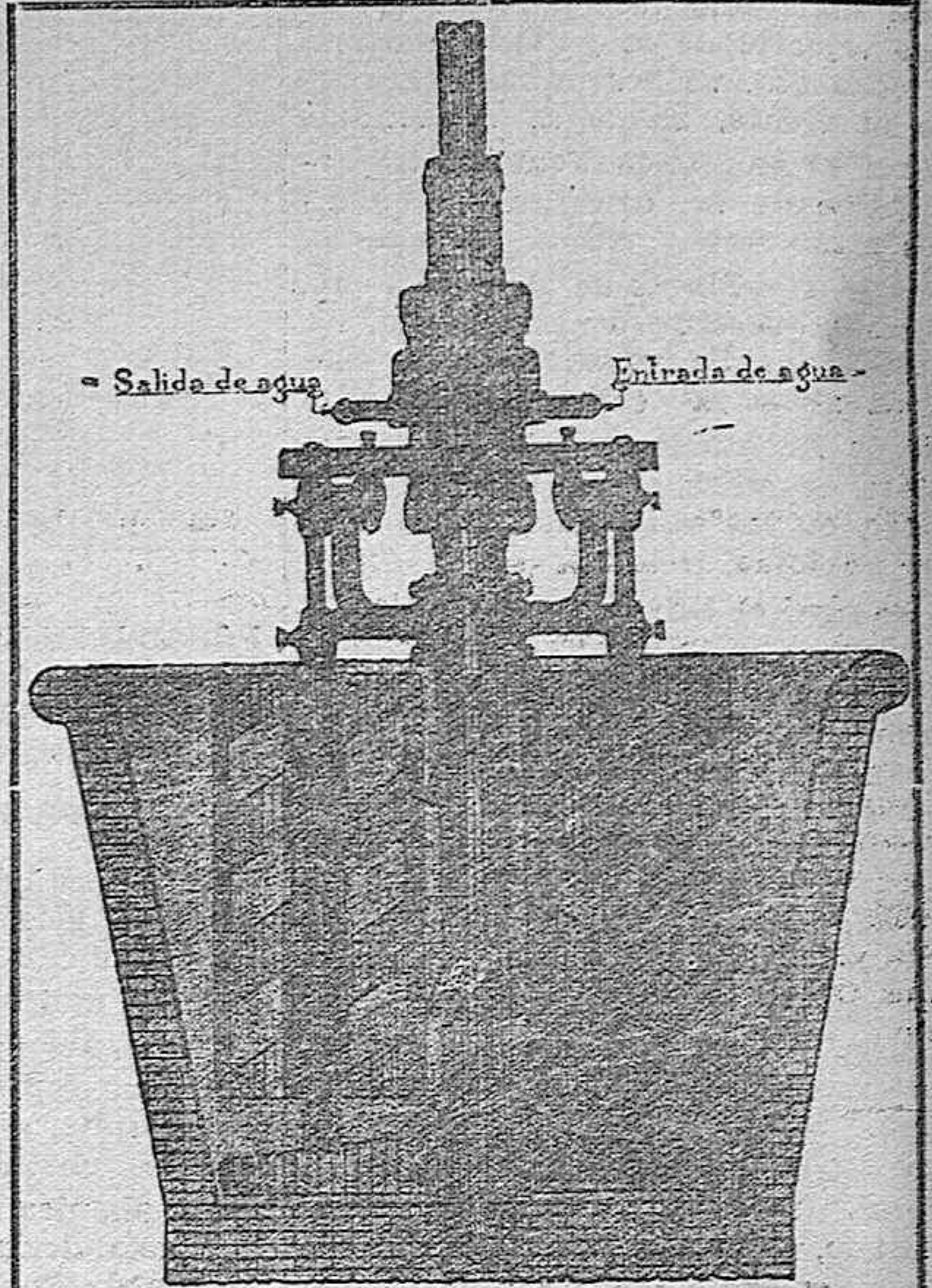
Una vista de mi batidora sin piedras y con dispositivo especial de calefacción en sus paletas y soporte central patente 131.064
