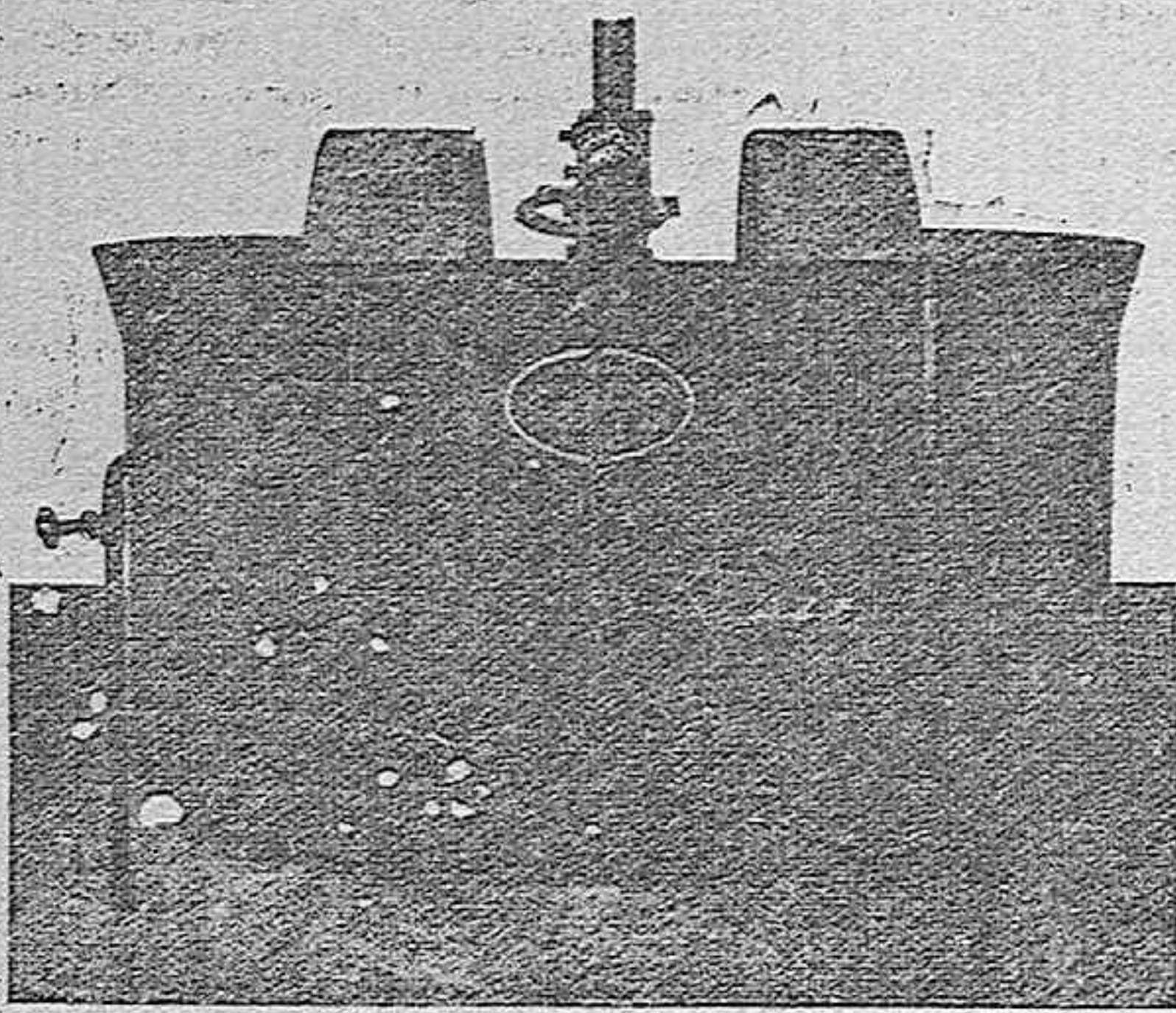
Vista de mi batidora-remoledora con piedras y envolvente de calefacción, patente 105.299.
