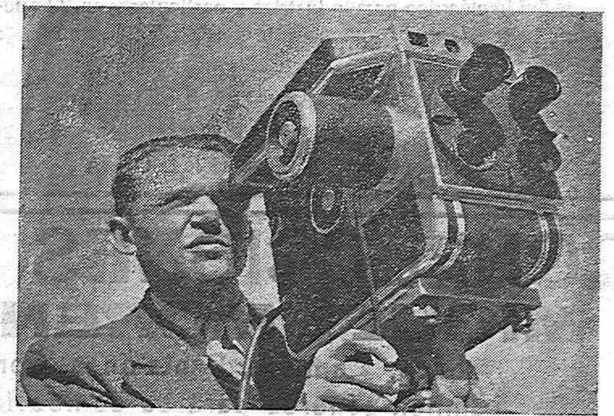
BERLIN.—EL "IKOPHON" ES EL PRIMER APARATO DE FORMATO PEQUEÑO DEL MUNDO QUE PUEDE IMPRESIONAR TONO Y FOTOGRAFIA EN LA MISMA CINTA DE PELICULA DE PASO ESTRECHO. ES LA PRIMERA CAMARA DE CINE SONORO PARA LOS AFICIONADOS.
