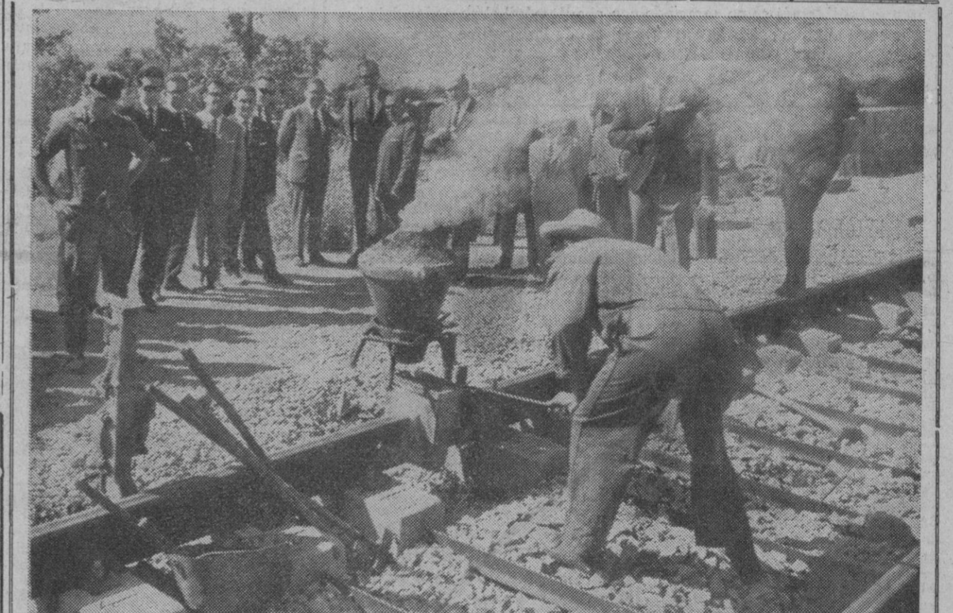
Miraflores (Madrid).—El ministro de Obras Públicas acompañado de personalidades de su Departamento, observa una soldadura de carriles durante su visita a las obras del ferrocarril Madrid - Burgos (Foto Europa Press)
