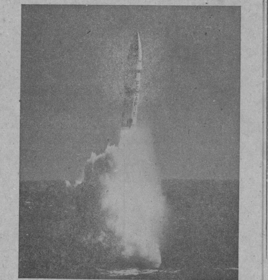
El Polaris A-3, tercera generación de los proyectiles lanzados desde submarinos atómicos sumergidos, entrará en funcionamiento a finales de 1964. Tiene un alcance de 4.600 kilómetros, unos 1.850 más que el modelo anterior, el A-2. Tanto el A-2 como el A-3, así como el anterior A-1 pueden ir armados de cabeza nuclear. Aquí vemos al A-3 en el momento de iniciar su trayectoria en el Campo Experimental de Tiro del Atlántico después de su lanzamiento desde el submarino atómico norteamericano "USS Andrew Jackson", estando éste sumergido.
