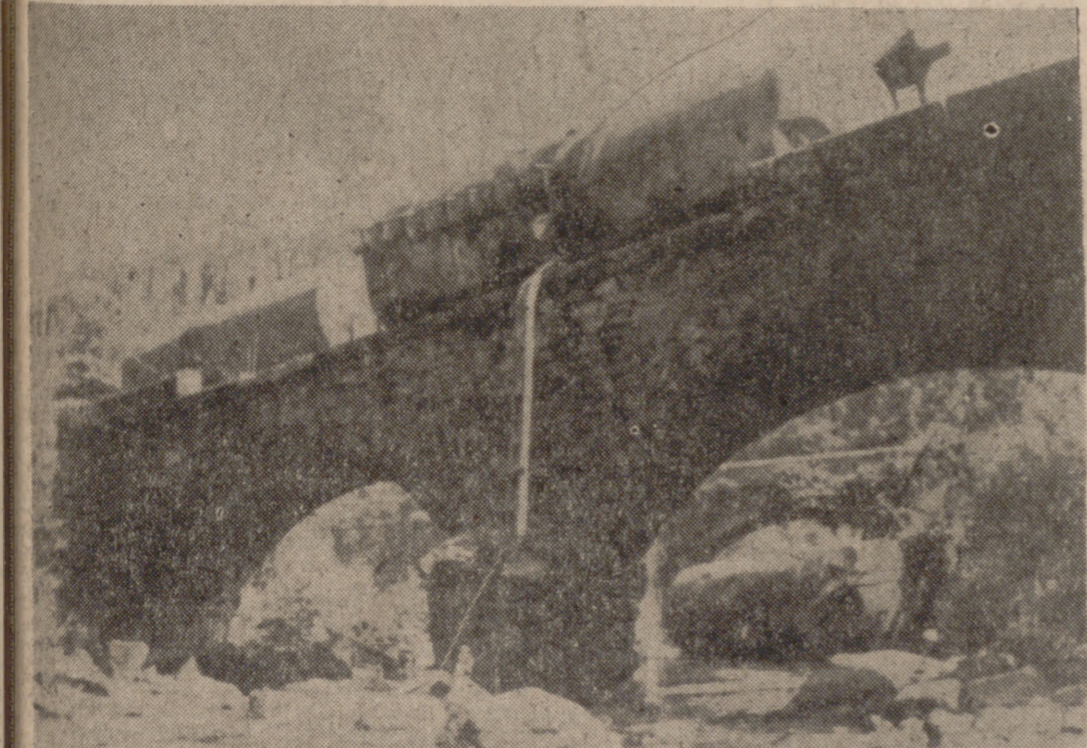
SANTANDER. — Un tren cisterna, compuesto por varias unidades, que transportaban combustible, descarriló en la línea Santander-Madrid, entre las estaciones de Molledo y Bárcena de Pie de Concha, a unos 45 kilómetros de Santander, en el llamado Puente del Rey. Uno de los vagones, que contenía 50.000 litros de gas-oil, se incendió. Otro de los vagones quedó al borde del río, derramándose los 63.500 litros de gasolina que transportaba. En la foto, un aspecto del lugar del accidente. (Telefoto Cifra Gráfica.)
