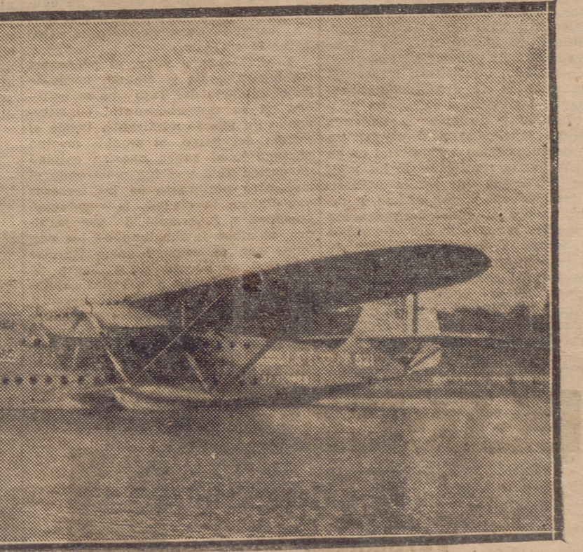
EL HIDROAVION GIGANTE "LIEUTENANT DE VAISSEAU PARIS", QUE POR CAUSAS DESCONOCIDAS HA SUFRIDO EN BURDEOS UN IMPORTANTE INCENDIO QUE LO HA DESTRUIDO CASI TOTALMENTE. LAS AUTORIDADES INVESTIGAN SOBRE EL SUCESO. — ARRIBA A LA IZQUIERDA EL TENIENTE DE NAVIO, PARIS
