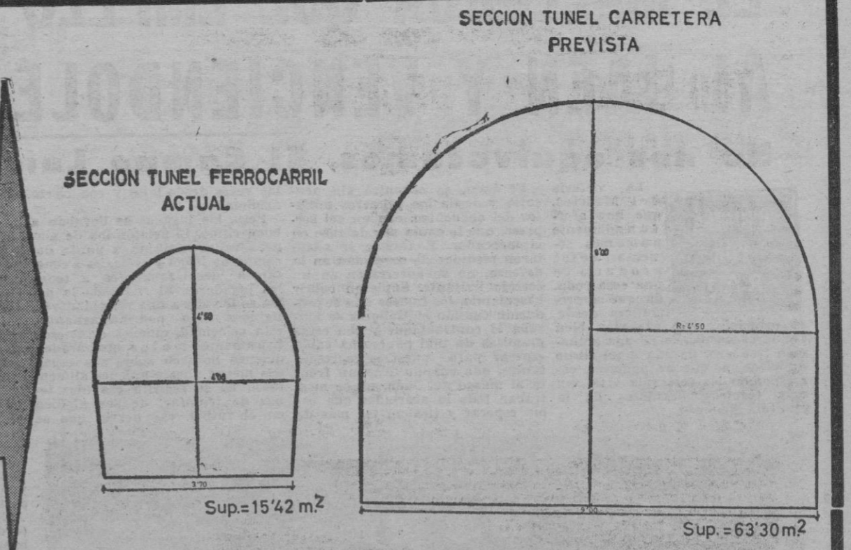
EL LECTOR PODRÁ ApreciAR A LA IZQUIERDA EL PLANO DE UNA SECCION VERTICAL DEL TUNEL EN SU ESTADO ACTUAL, A LA DERECHA, TAL COMO QUEDARÍA EL DE LA CARRETERA COMO SE VE, TENDRÍA QUE SER AMPLIADO A NUEVE METROS DE ANCHO Y OCHO DE ALTURA.
