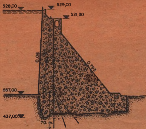
PRESA DE MEDIANO (EN CONSTRUCCION)
