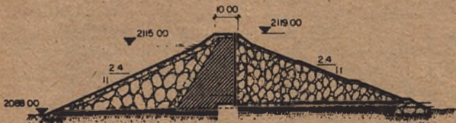
PRESA DE I.P. (En construcción).
