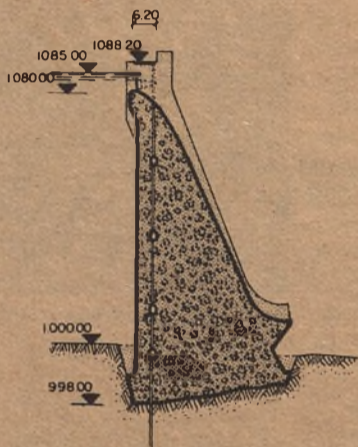
PRESA DE BUBAL
