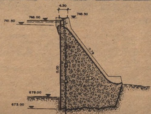
PRESA DE VADIELLO
