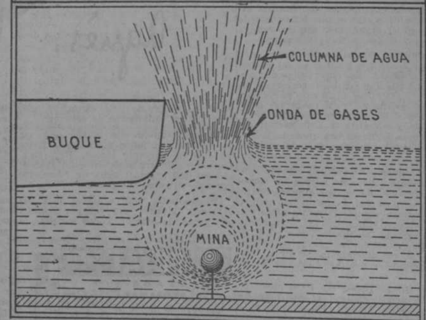
Cómo se produce una explosión submarina
