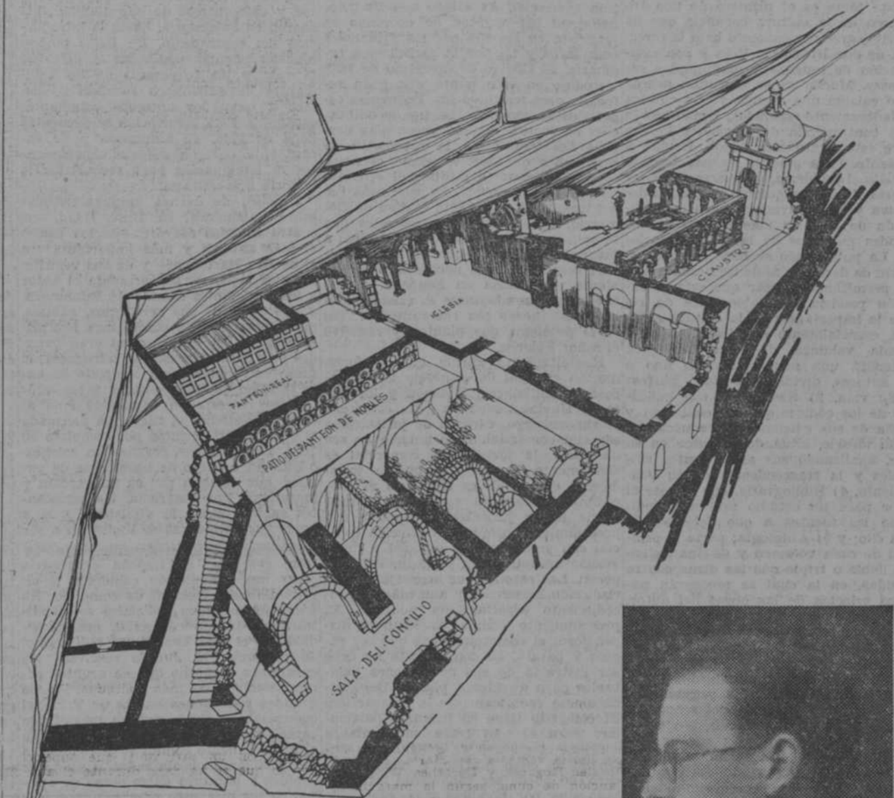
Plano inédito del Monasterio restaurado. (Arq. señor Iñiguez)
