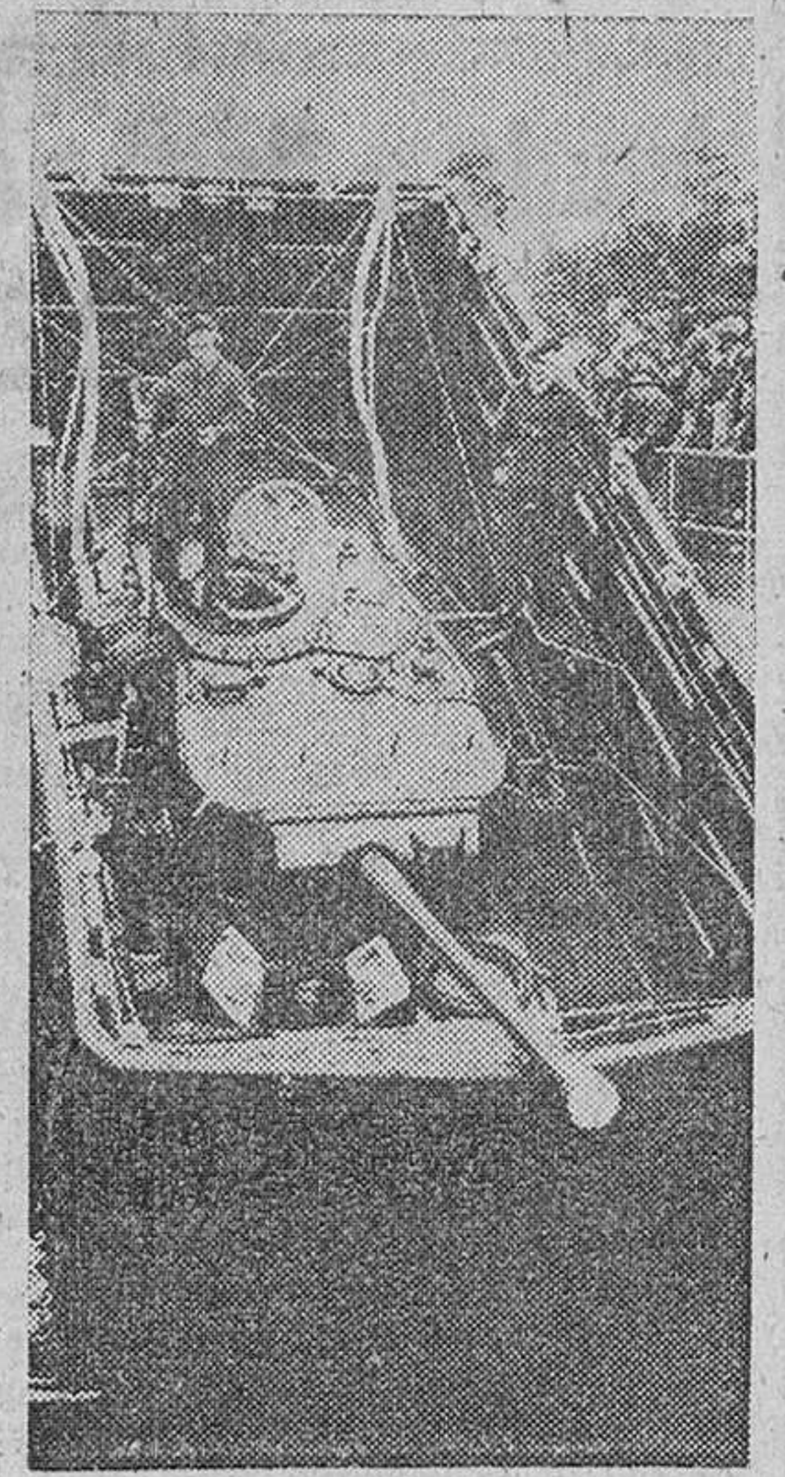
Agregados militares y técnicos de numerosos países, incluidos Rusia y Alemania, han presenciado en Surrey una demostración con un tanque británico "Centurión" de cincuenta toneladas, que flota sobre el agua sin necesidad de cerrar las escotillas. En esta situación puede seguir disparando. — (Foto Gil del Espinar)
