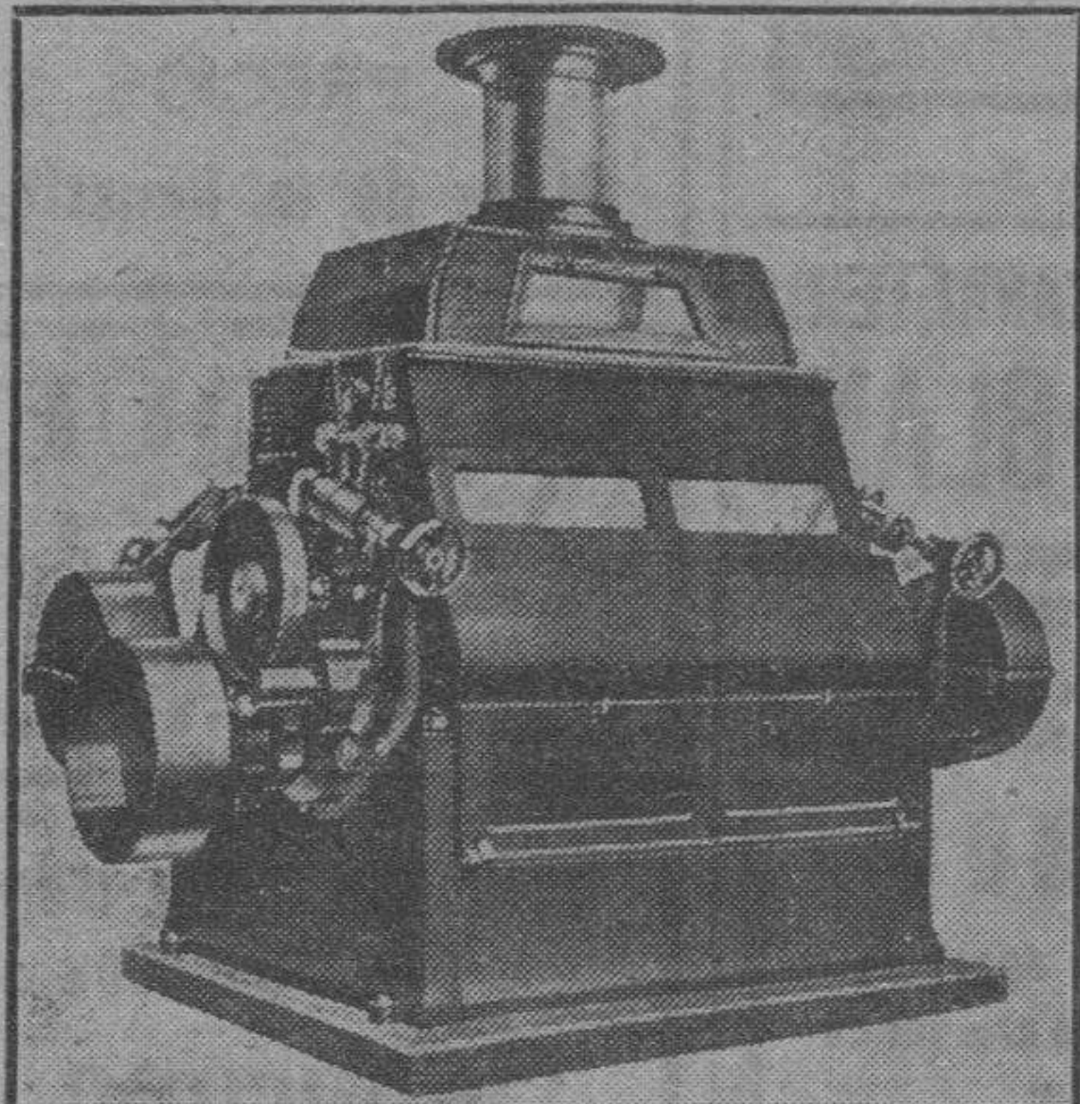
Molino diagonal de cuatro cilindros
