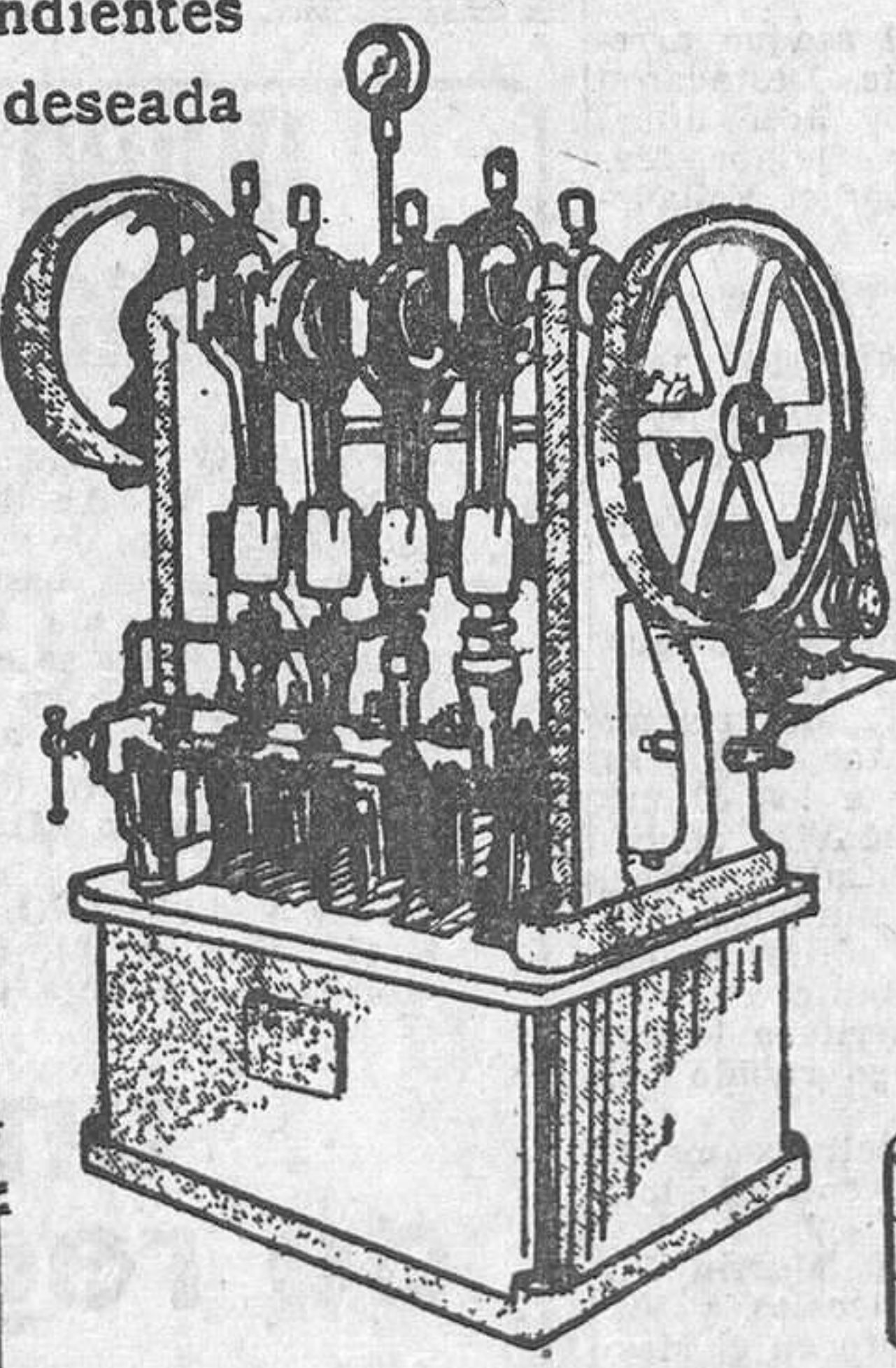
Prensa monobloque todo acero Vagonetas sin carriles
