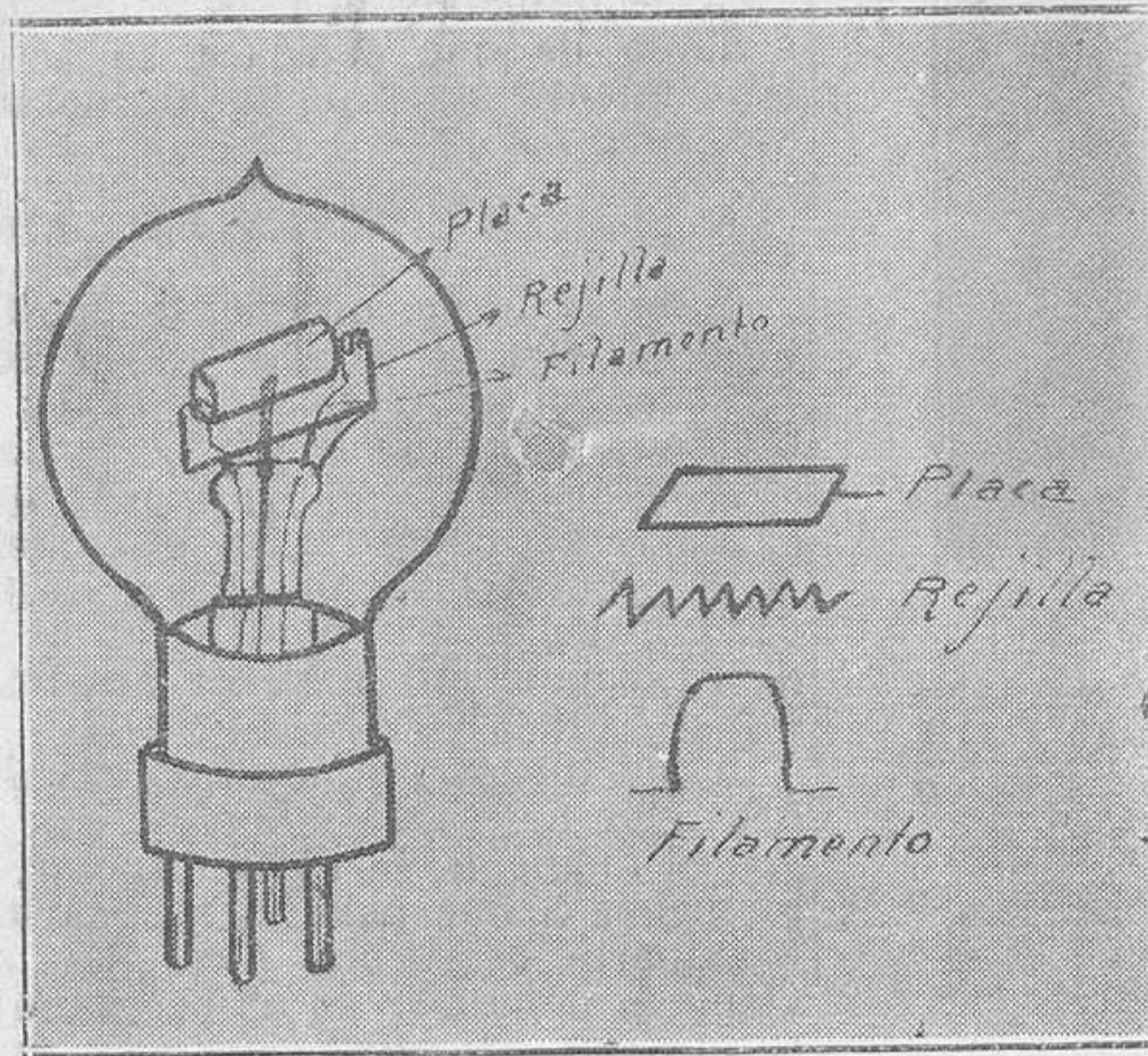
Lámpara de tres electrodos, forma real y dibujo en esquema.
