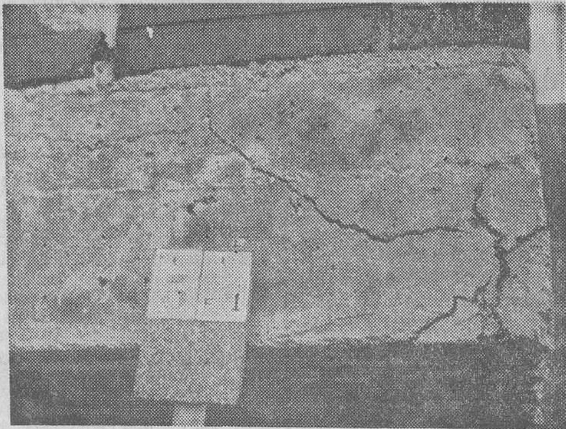
La fotografía presenta una muestra del agrietamiento en el edificio que estaba destinado a ser el futuro colegio de subnormales de Mataró. (Foto Tomás Manent.)
