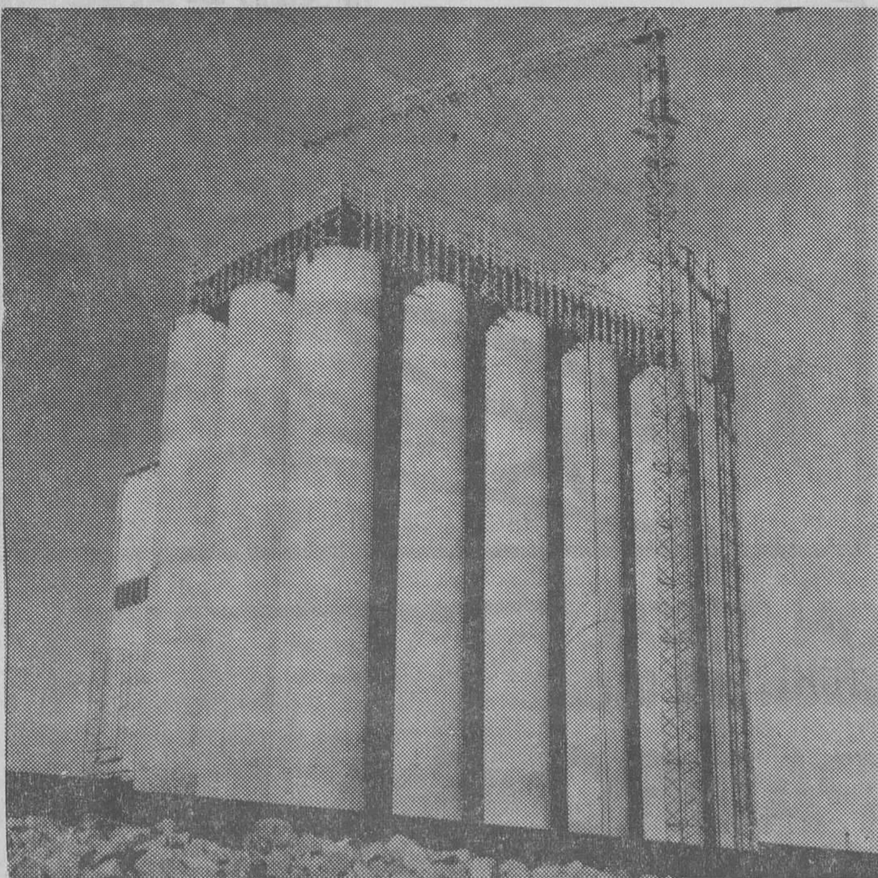
Estado de las obras de construcción de la nueva factoría de «Piensos Equilibrados C.I.A.» que se está construyendo en Vilafranca del Penedés. Los silos para cereales que se contemplan en la fotografía tienen capacidad para 7.680 toneladas. Las obras dieron comienzo en septiembre de 1966 y estarán terminadas el próximo mes de marzo
