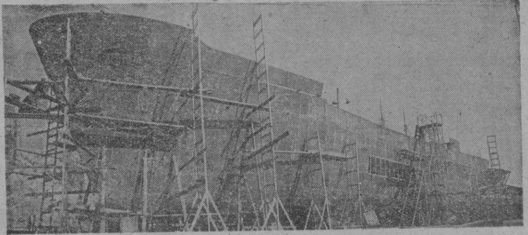
El primer barco de casco de acero construido en Mallorca, en la grada de los «Astilleros Palma S. A.» — (Foto Juanet)
