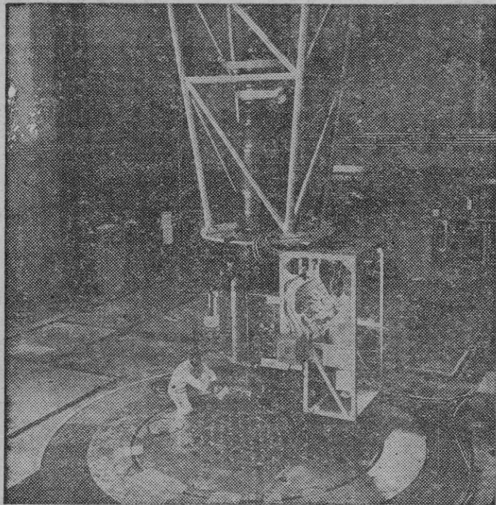
Los técnicos norteamericanos comprueban el funcionamiento de una gigantesca cámara de plomo que sirve para cargar uranio dentro del núcleo de un reactor de energía atómica que se encuentra a gran profundidad bajo el suelo.
