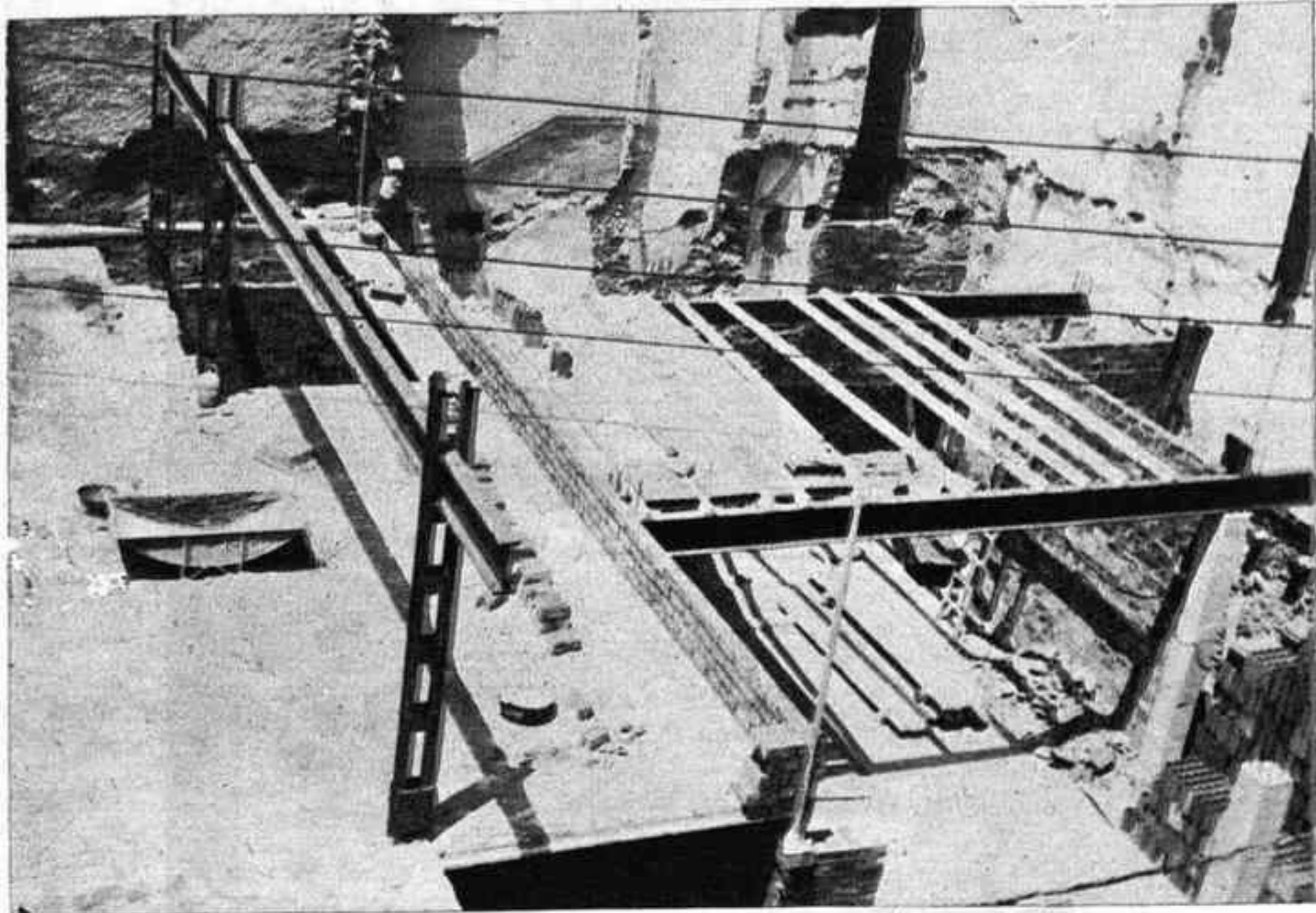
Estructuras MIXTAS
