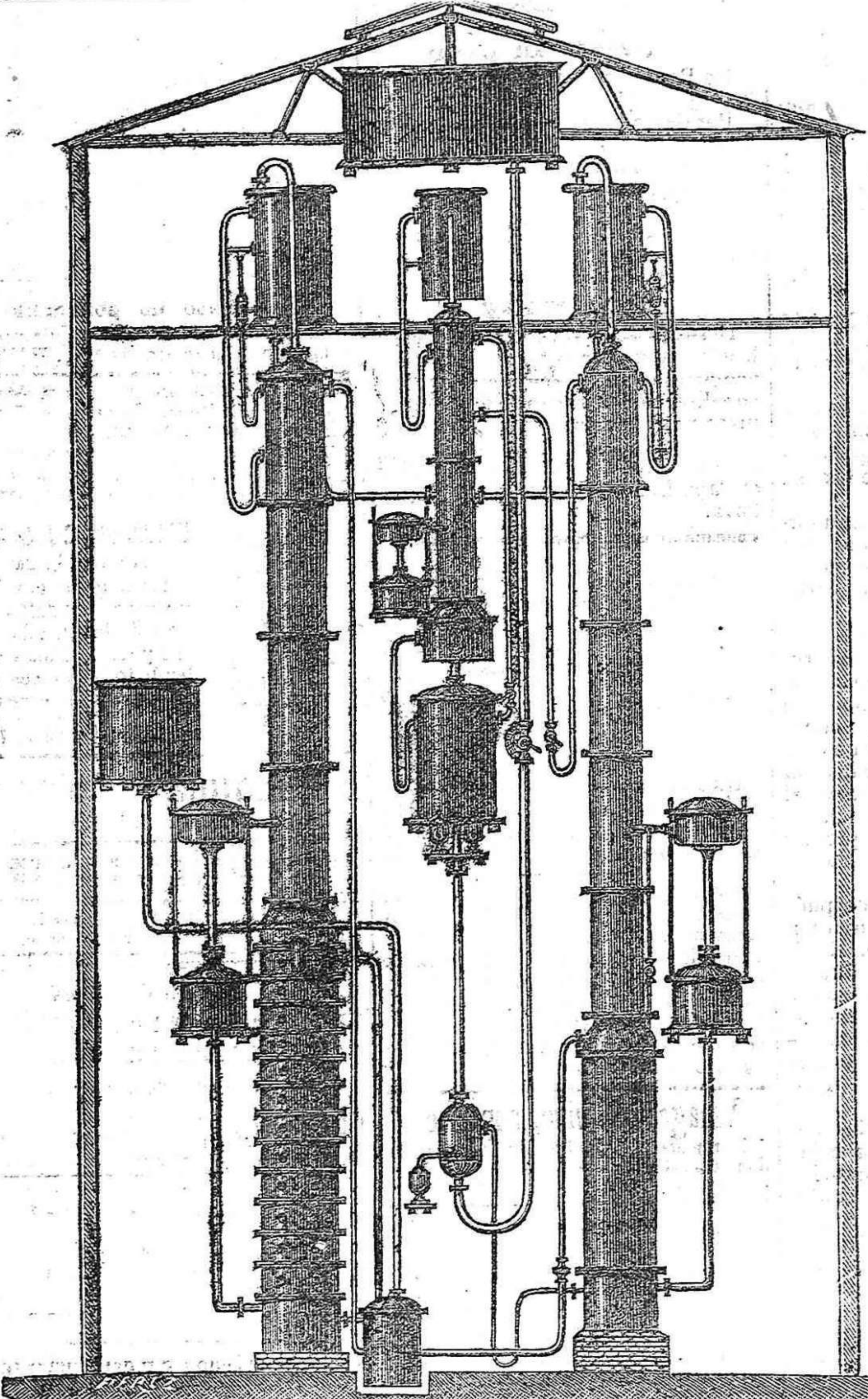
RECTIFICADOR AUTOMÁTICO CONTINUO SISTEMA A. M. FROMENT, CON REAL PRIVILEGIO
