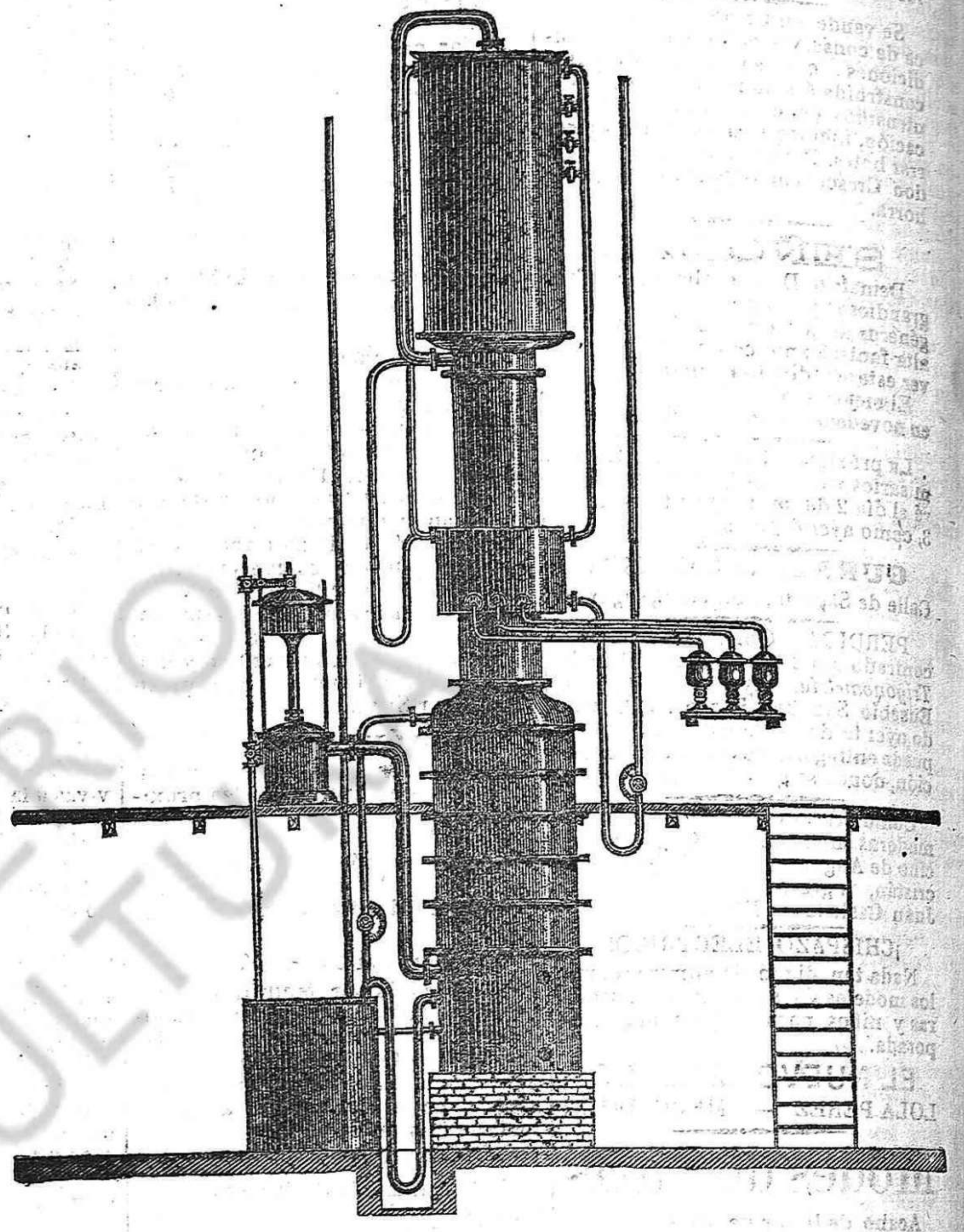
DESTILADOR DEPURADOR CONTINUO O DISCONTINUO A FUEGO DIRECTO Ó A VAPOR =PERFECCIÓN= sistema A. M. FROMENT
