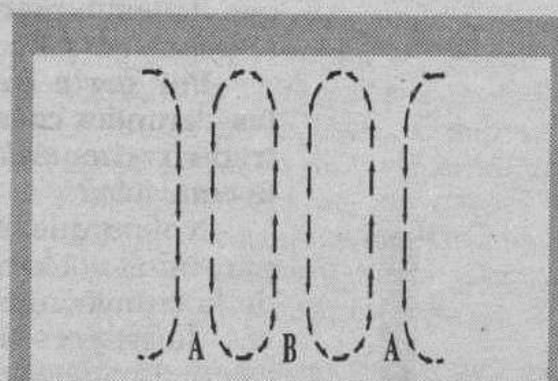
Sección de anticiclones y bajas presiones
