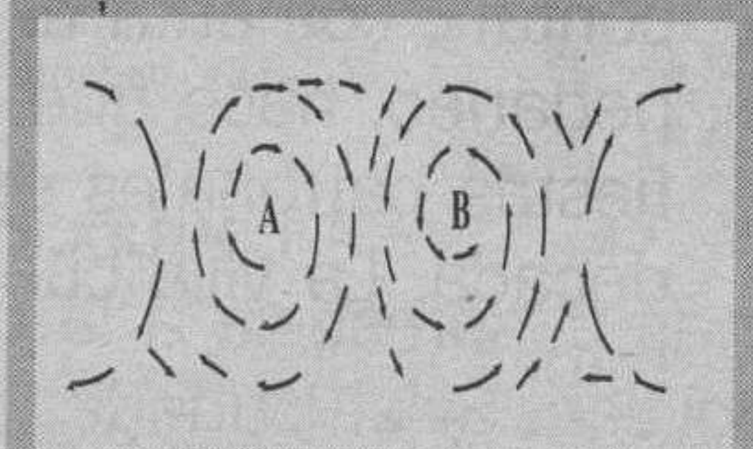
Plano horizontal de altas y bajas presiones
