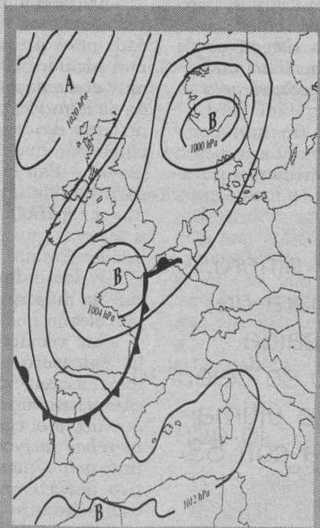
Mapa del tiempo en el que quedan reflejadas altas y bajas presiones además de un frente ocluido.
