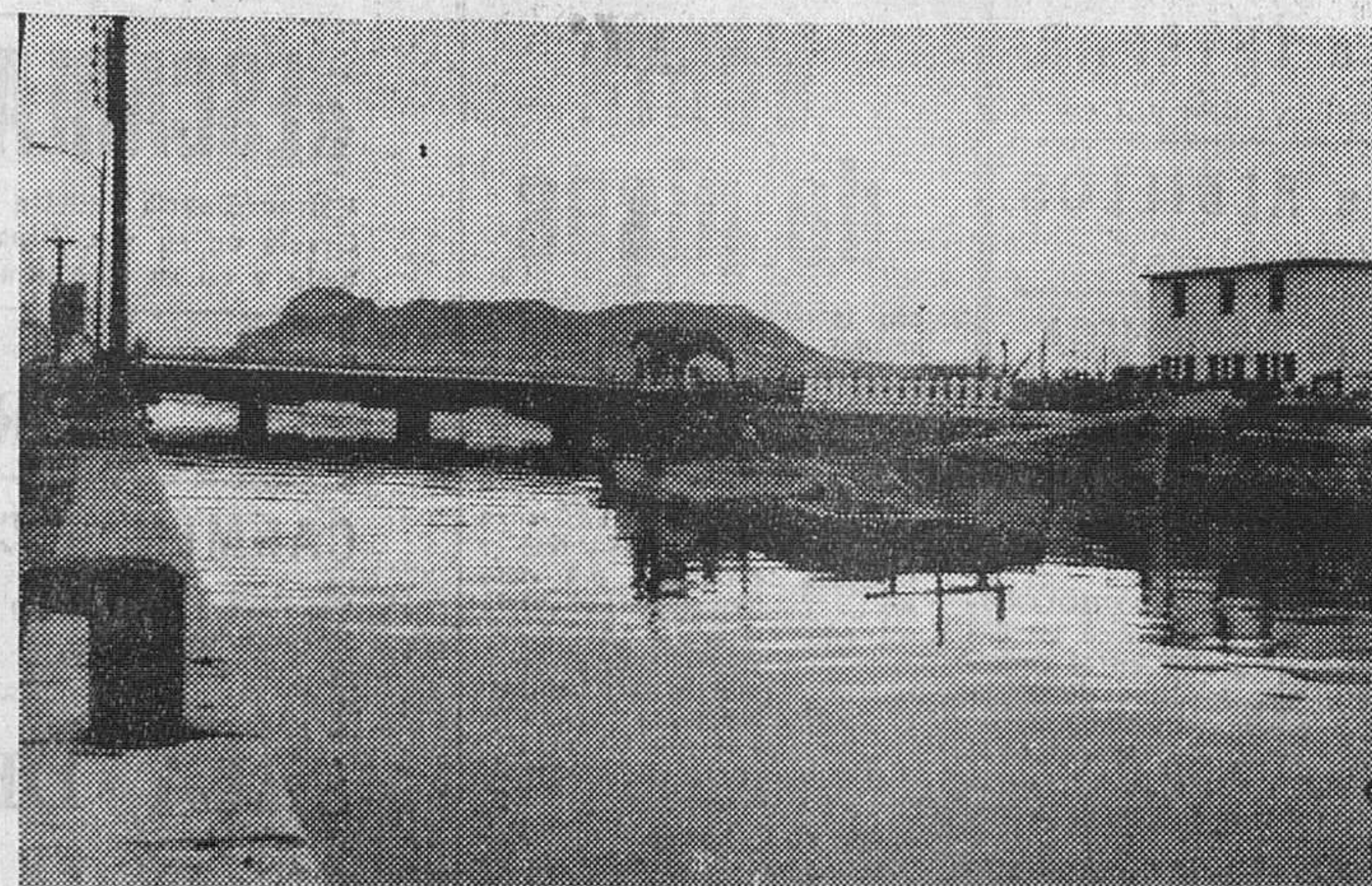
Se construye actualmente un nuevo puente sobre el río La Miel junto a Algeciras, sobre el que pasará la autopista Cádiz-Málaga. La fotografía recoge un aspecto de las obras con el perfil del Peñón al fondo. — (Foto FIEL)
