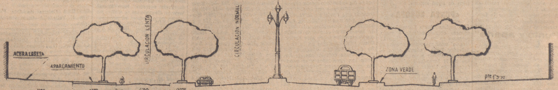
Perfil transversal de las obras de transformación de andenes y nuevas calzadas del Paseo de Zorrilla. En el dibujo se ve con suficiente claridad en lo que han de consistir los cambios. De izquierda a derecha, acera de siete metros, como mínimo, con pavimento de loseta hidráulica; abarcando la primera hilera de árboles, una calzada para aparcamientos en batería y parada de taxis, de 4,75 m.; calzada de circulación lenta, destinada a servicios del vecindario, de seis metros; una modesta zona verde que abarca las filas de arbolado interior; calzada de circulación normal para tres vehículos en una misma dirección, farolas y división central con setos; repetición del dispositivo en sentido inverso. Pendientes de las aceras, 15 ‰. (Croquis de Casado.)
