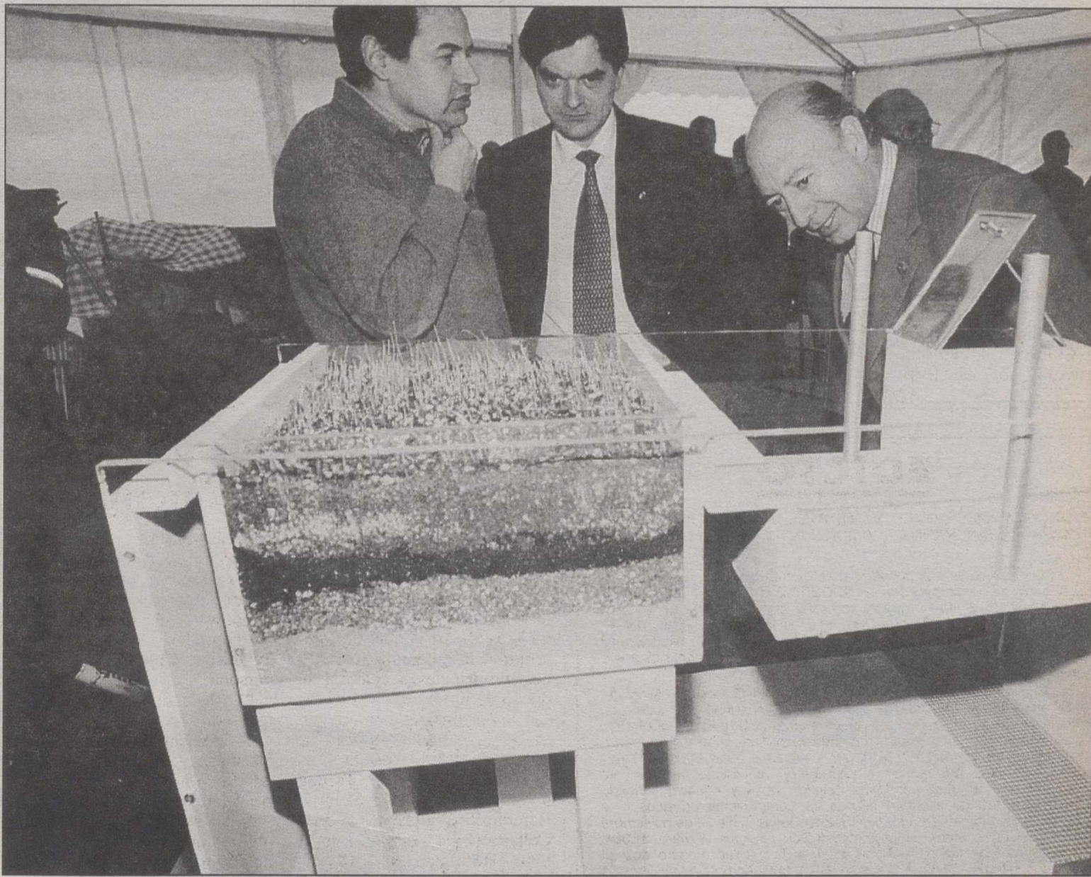
Modelo a escala de la Estación de Lisimetría instalada en la finca de Las Tiesas.
