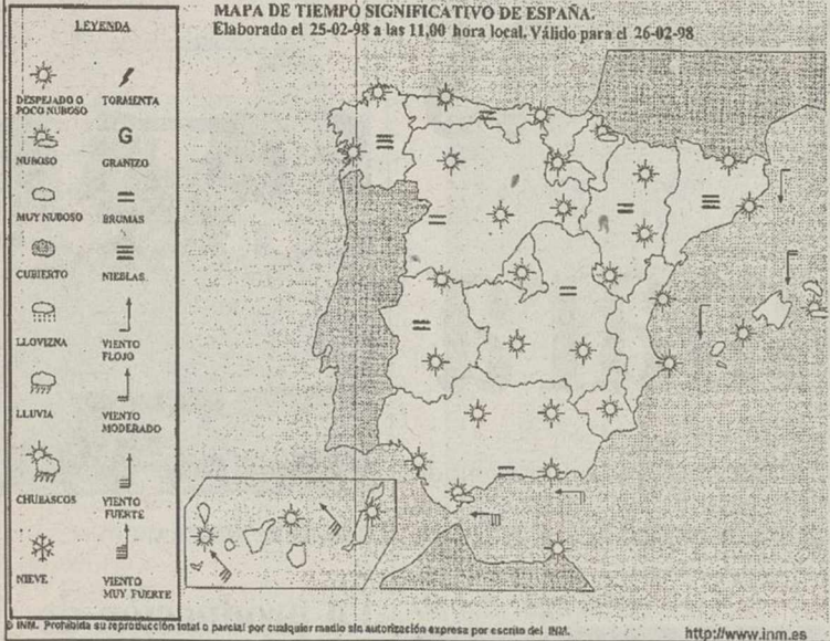
Ministerio de Medio Ambiente Instituto Nacional de Meteorología MAPA PREVISTO DE SUPERFICIE VALIDO 26-2-98 A 12 UTC, IV
