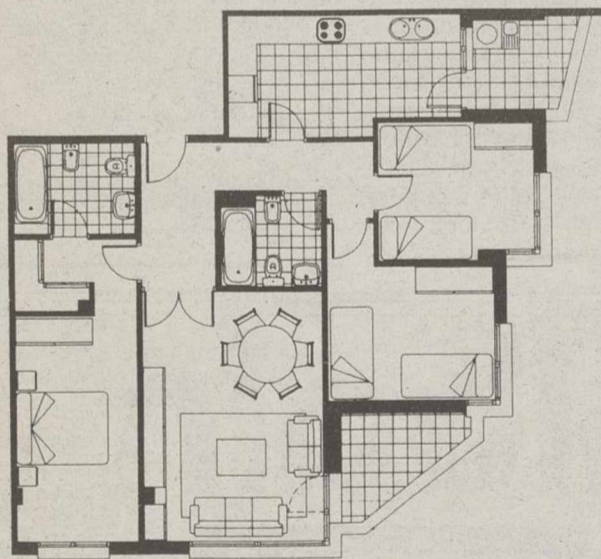
Detalle Piso 3 dormitorios Superficie útil 91,79 m 2
