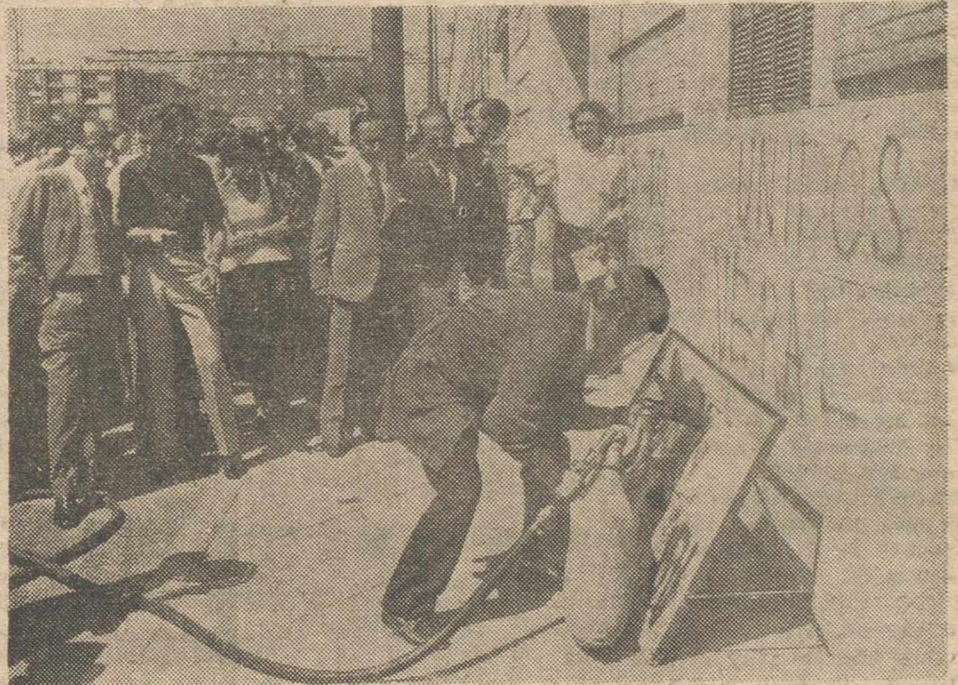
MADRID.— El Ayuntamiento de Madrid ha presentado sus nuevos equipos para borrar las pintadas en los edificios de la ciudad. Después de numerosas investigaciones han conseguido un equipo compuesto por un vehículo-camión ligero, un compresor rotativo, un carrete manguera y el depósito de granalla. Asistieron a la presentación de este equipo el gobernador civil de Madrid, señor Rosón, y el alcalde, señor Alvarez, entre otras personalidades.— (FOTO EUROPA PRESS).
