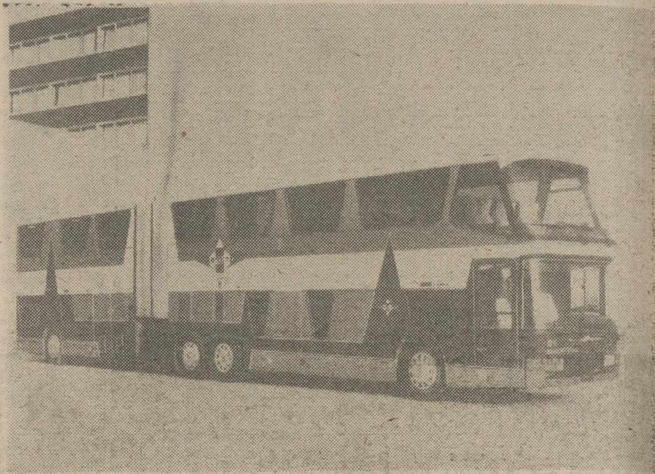
STUTTGART (DaD). — El mayor bus-hotel del mundo ha sido construido en unos talleres especiales de la República Federal de Alemania. El "Car-o-tel" (foto) dispone de 8 cabinas de dos literas, WC, ducha, aire refrigerado, cocina, bar y de una "sala panorámica" ubicada sobre el conductor. — (Foto: DaD/Auwärter).
