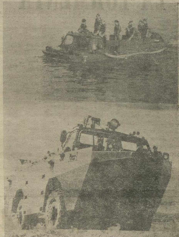
MADRID. — Dos aspectos del Transporte Anfíbio 3.550 que con destino a la Infantería de Marina, ha sido diseñado para la utilización continua en zonas de mar y playa en desplazamientos constantes. Tiene un probada manejabilidad y consigue por carretera una velocidad de 100 kilómetros a la hora. — (Foto EUROPA PRESS).
