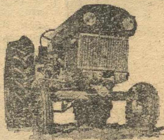
R-500 B - 52 CV HMA Con éste basta para hacerlo todo.
