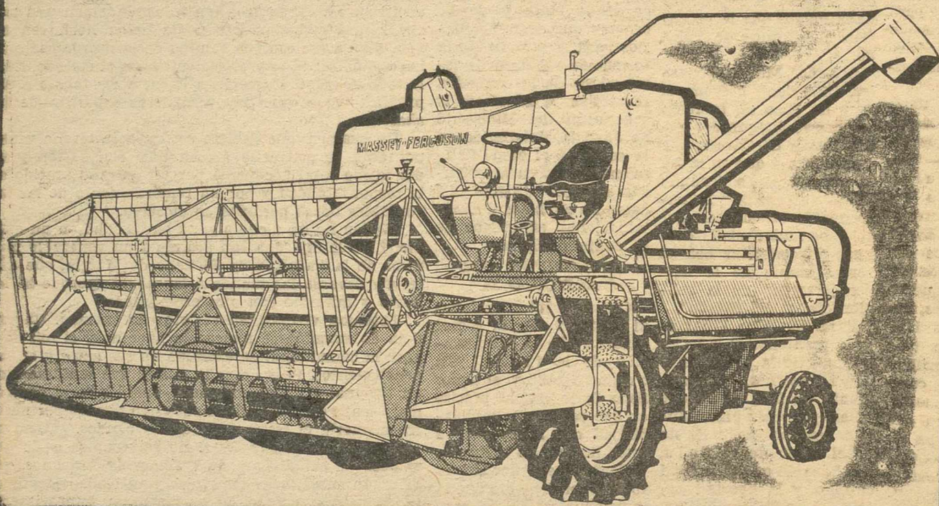
LA MF 87-12 MIXTA DISPUESTA PARA TRABAJAR CON TANQUE
