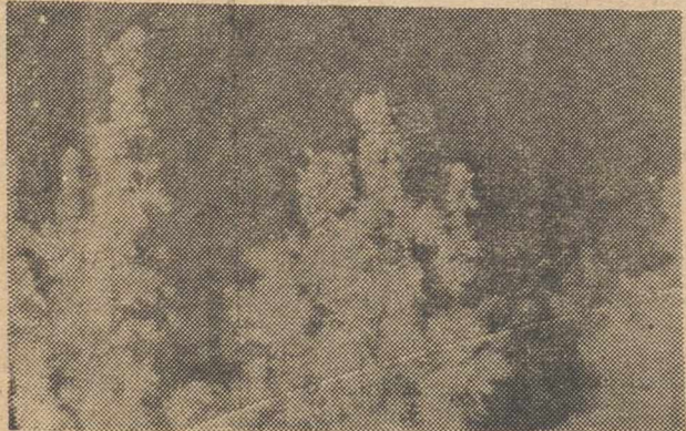
Concreciones arracimadas de la cueva del Nispero (Burgos).—Foto: R. Plá.
