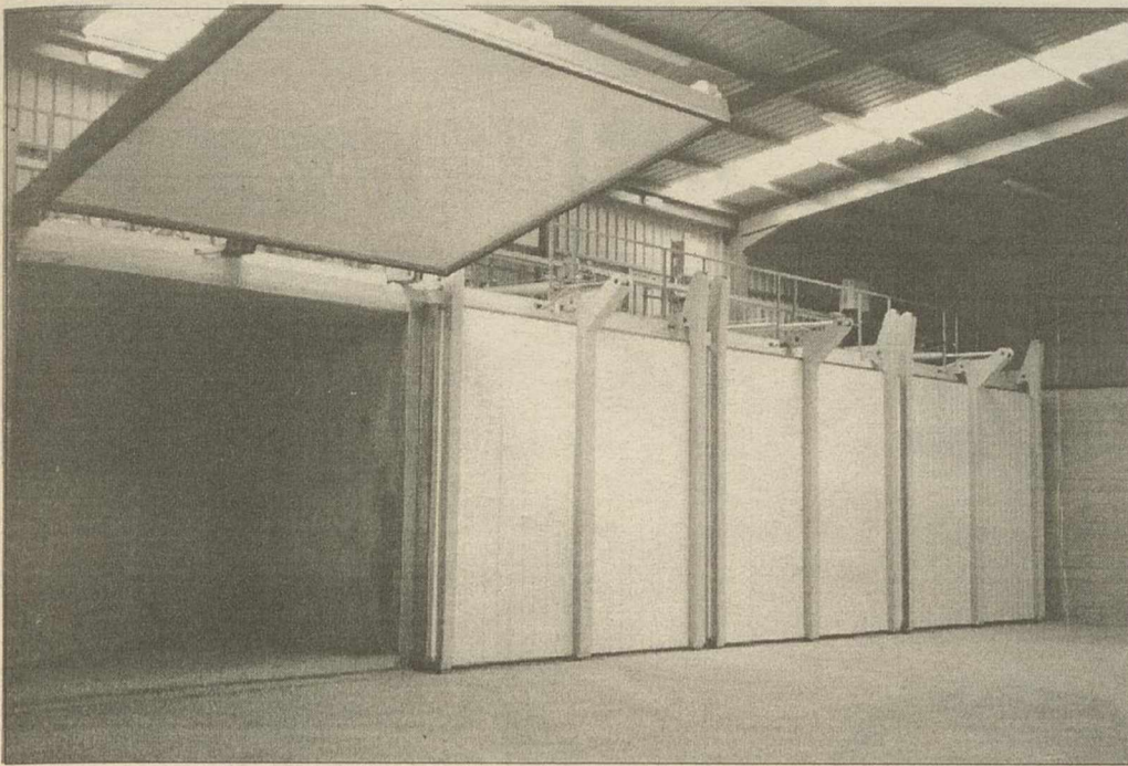
Boxes de la planta de reciclaje de Almagro donde se realiza el proceso de fermentación.
