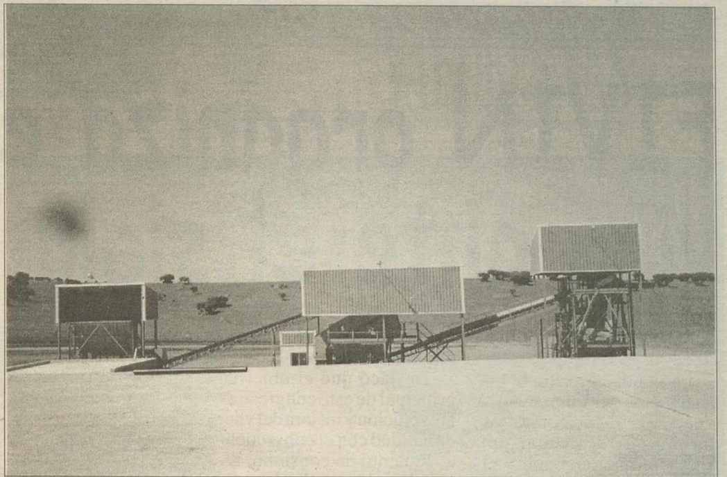
Cadena de filtros para el afino y resultado final del compost.
