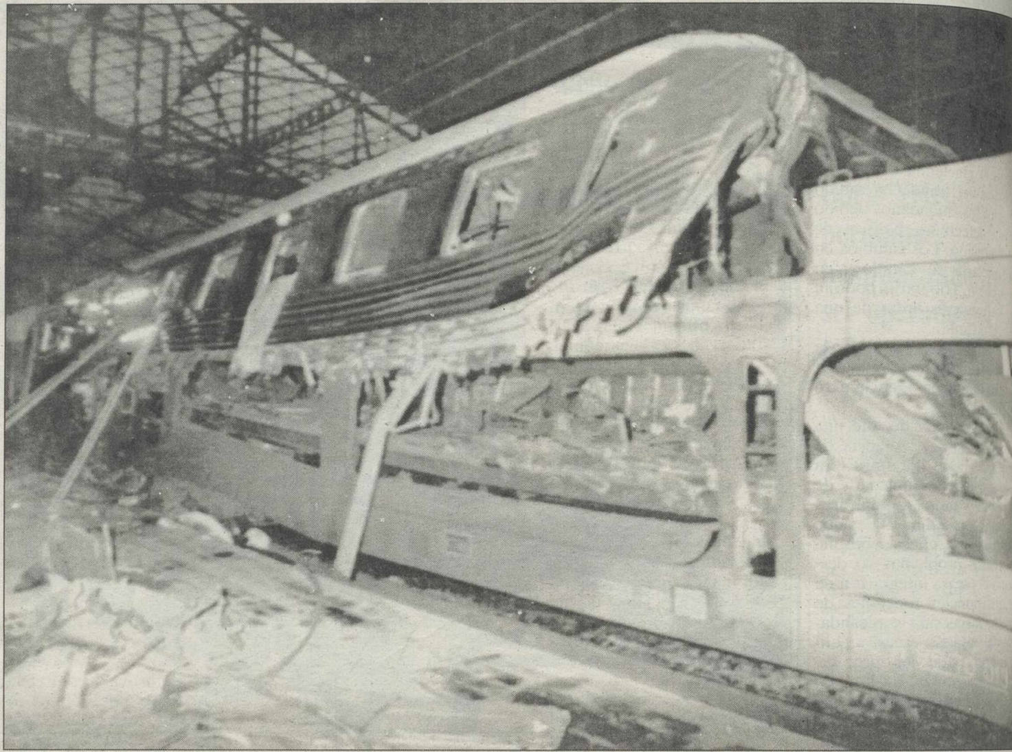
El Correo 421, que cubría el recorrido entre Madrid y Galicia, colisionó de forma fatal con una máquina que hacía maniobras en un túnel.
