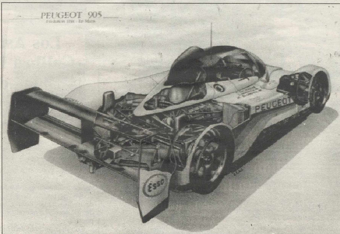
Radiografía del coche campeón, en su versión "Le Mans".
