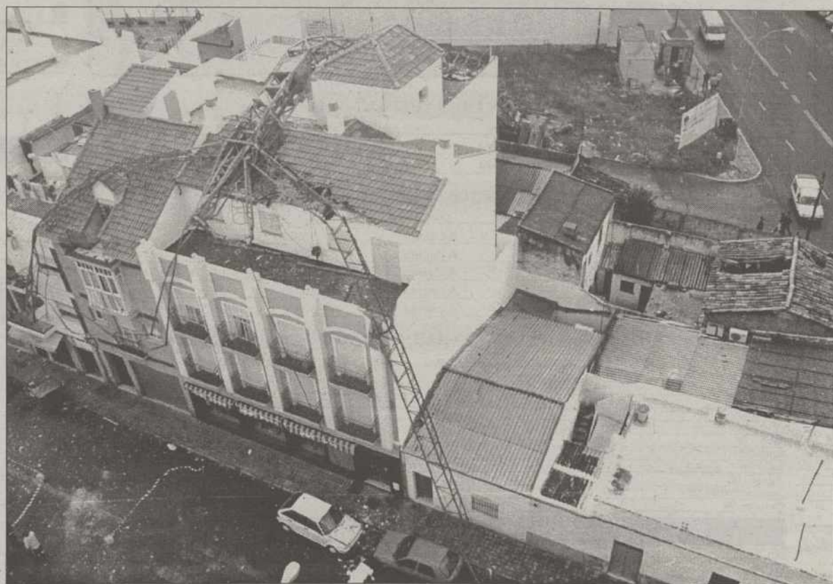
Desplome de una grúa de obra en un barrio de Sevilla.
