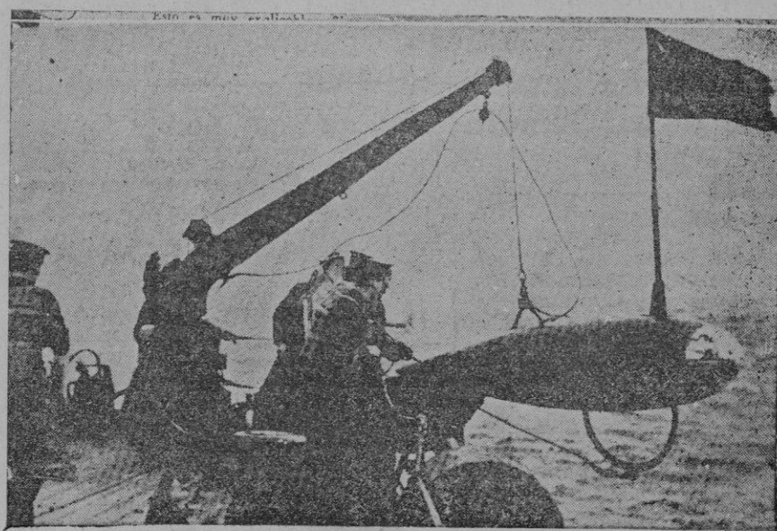
Los dragadores ingleses, en el mar del Norte, colocan en el agua flotadores que, unidos entre sí por un cable provisto de cortadores, limpian de minas los mares
