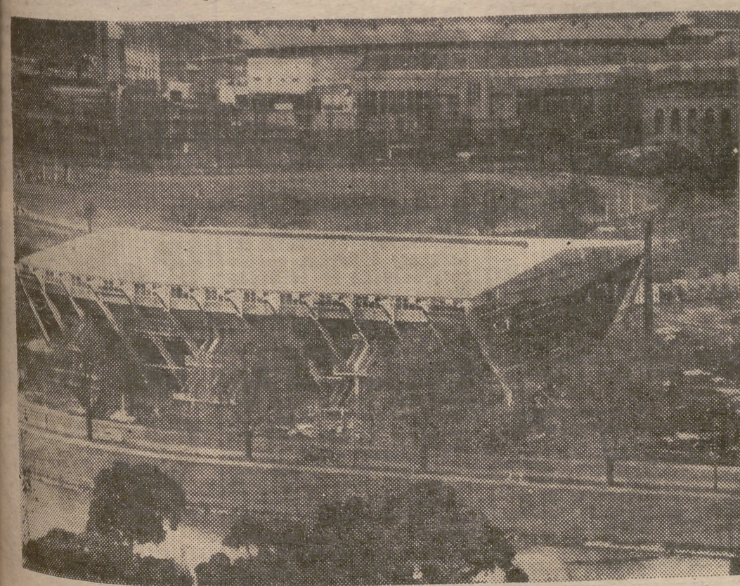
Una vista de la preparación y construcción del estadio piscina para los Juegos Olímpicos que tiene cabida para 4.000 personas. Al fondo vemos otro estadio, el de Cricket Ground, que tiene capacidad para 110.000 personas (Foto Keystone Nemes)
