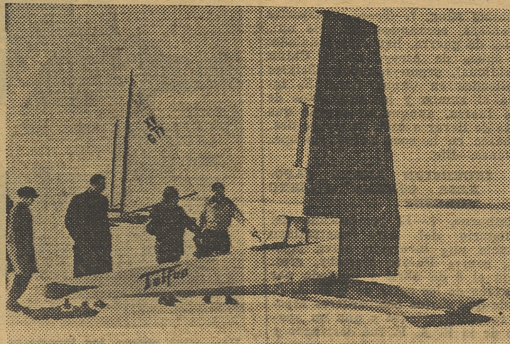
Nueva construcción de trineo a vela, capaz de alcanzar 200 kilómetros por hora, en una de sus pruebas recientes. (Foto Orbis.)
