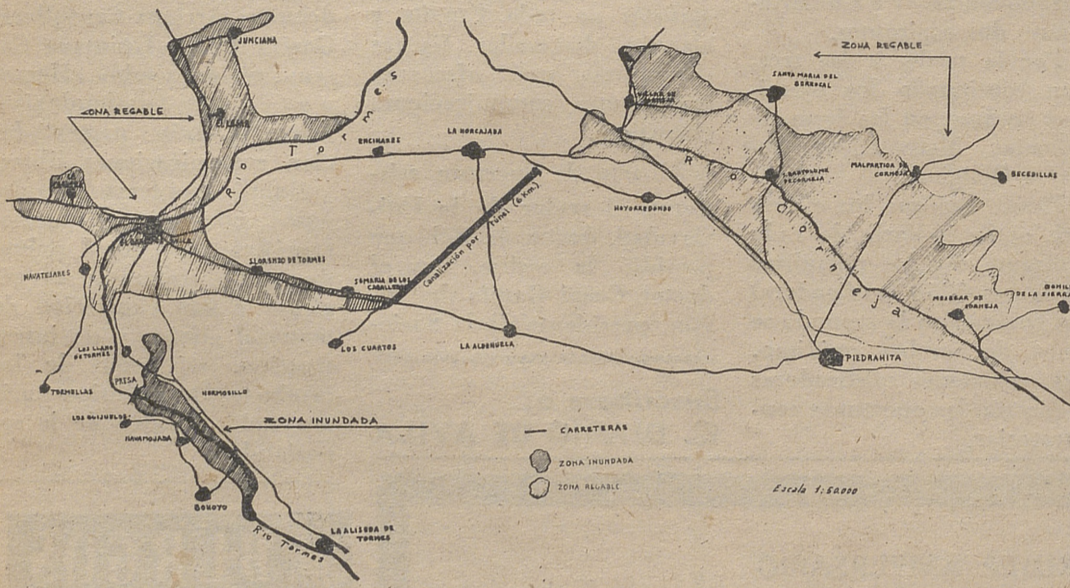
PLANO GENERAL DEL PROYECTO DE NUEVOS REGADIOS EN 7.500 H.A. DEL VALLE DEL CORNEJA
