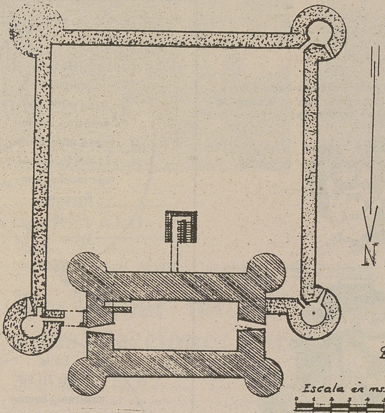
Castillo de Fuensaldaña, sede de las Cortes actuales. Planta.
