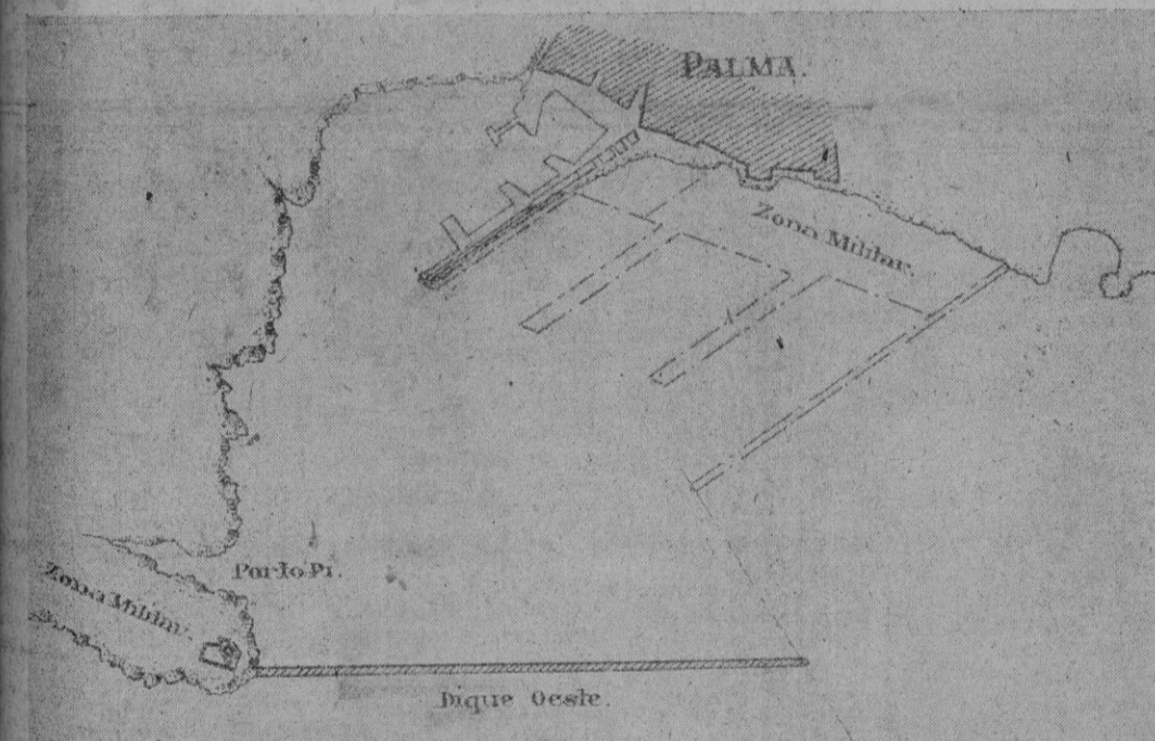
Plano del actual puerto de Palma, con el nuevo Dique del Oeste que arrancará de la punta de San Carlos. La línea que pasa por la punta del Dique del Oeste indica la dirección de los vientos dominantes en nuestra bahía.
