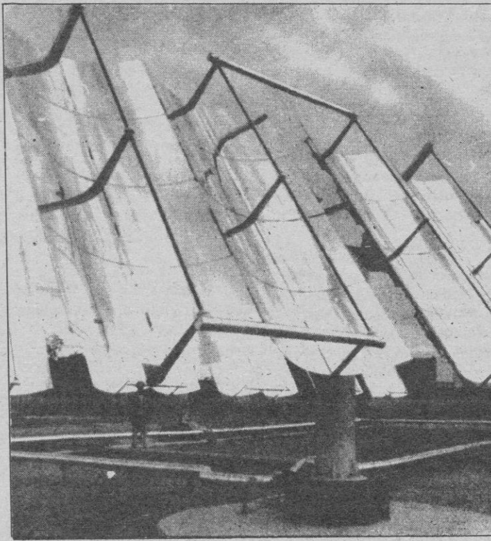
El ministro de Industria, Ignacio Bayón, inauguró ayer, en el término de Getafe (Madrid), una «granja solar» de experimentación y ensayo, una de las primeras en su género en Europa. La planta, construida de forma conjunta por Auxini y la empresa alemana federal MAN, dispone de una superficie de 580 metros cuadrados de colectores y una capacidad de producción de 250 kilovatios térmicos. La «granja solar» tardó tres años en construirse y costó quinientos millones.—(Foto Efe)
