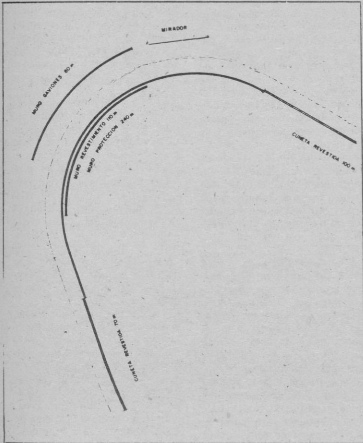
Un detalle del plano de la obra a realizar, si nos situamos en la carretera con dirección de Segovia a la Lastrilla se aprecia la situación de los muros de contención.
