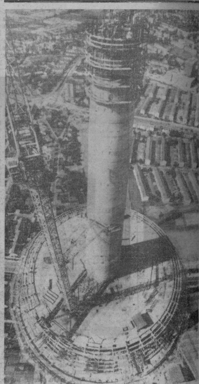
Vista aérea de las obras de construcción de la torre de Fráncfort del Meno (República Federal de Alemania), de 295 metros de altura y que estará terminada en la primavera del año 1979. Una vez montadas las antenas, la torre medirá 331,14 metros. Es la cuarta torre del mundo en lo que respecta a altura y la edificación más alta de la República Federal de Alemania. Pesa 50.000 toneladas y su construcción está presupuestada en 105 millones de marcos.
