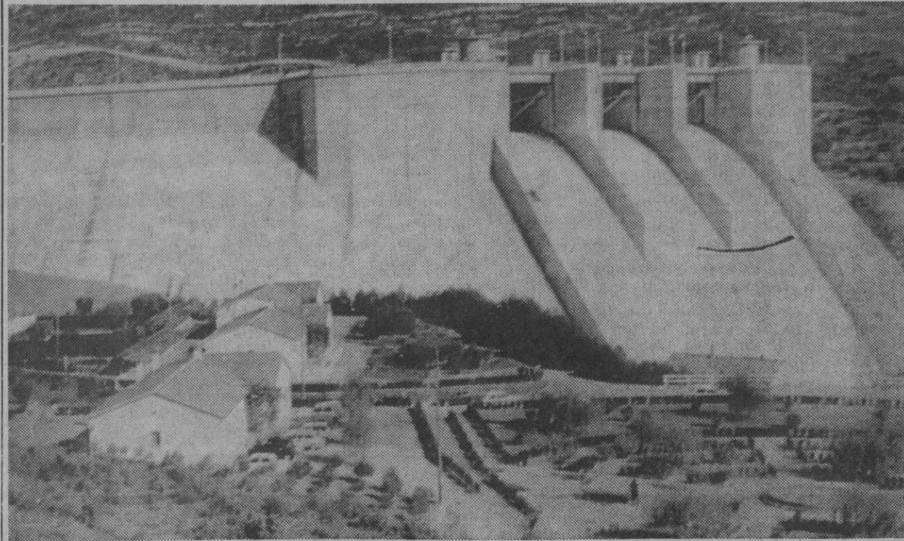
El Grado (Huesca).—Esta es la presa del pantano de El Grado, que ha sido inaugurada por los ministros de Obras Públicas e Industria.—(Telefoto E. Press)
