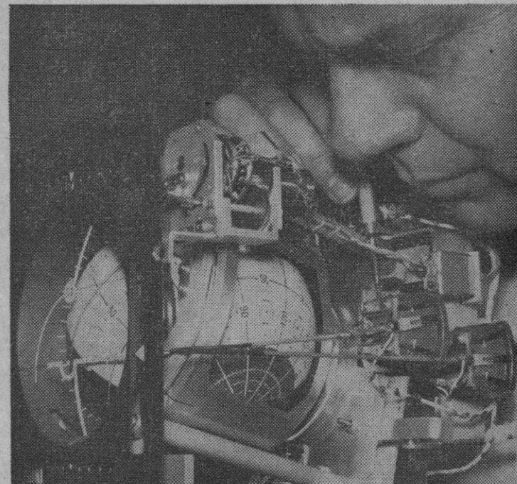
Un técnico de la fábrica Honeywell, en Minneapolis, opera en un indicador de posición de vuelo, diseñado para dar a los futuros astronautas del Apolo información de navegación durante los vuelos espaciales. La esfera muestra la posición del vehículo espacial Apolo en relación con sus varias órbitas. Unas agujas blancas indican las desviaciones de posición. El aparato está provisto de mandos manuales por si el equipo automático falla
