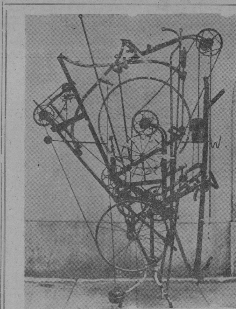
Este artefacto en forma de arpa es un excelentísimo reloj construido con seis bicicletas, el pie de una mesa, la cadena de un "water" y otras piezas más, por Joseph Heeb, de Ginebra, en 300 horas de paciente trabajo. La rueda grande superior, marca los minutos, y la pequeña, central, las horas.—(Foto Fiel.)
