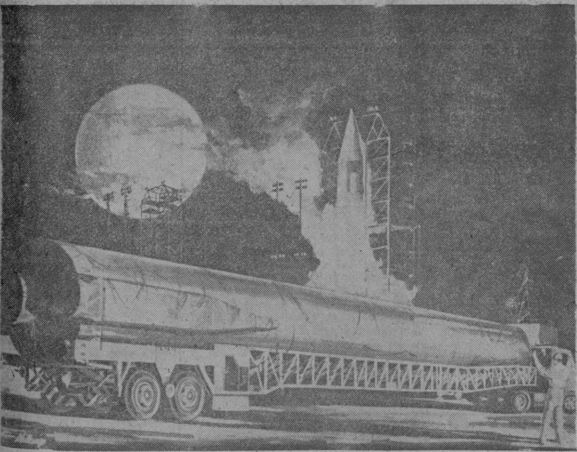
He aquí un aspecto general del largo remolque que conducirá los cohetes Atlas Centauro desde California hasta la estación de lanzamiento de Cabo Kennedy. El remolque ha sido especialmente diseñado para poder ser transportado por gigantes aviones de carga en el viaje hasta el lugar del lanzamiento. Una de las cabinas de la dirección puede verse inmediatamente delante del juego trasero de ruedas.—(Foto Fiel)
