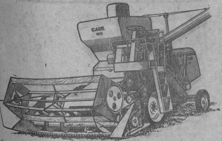
CASE Mod. 600 automotriz. Coschadora americana, 4 m. de corte. Motor «Case» 188, diesel 56 c. v. Crédito Agrícola y grandes facilidades de pago.
