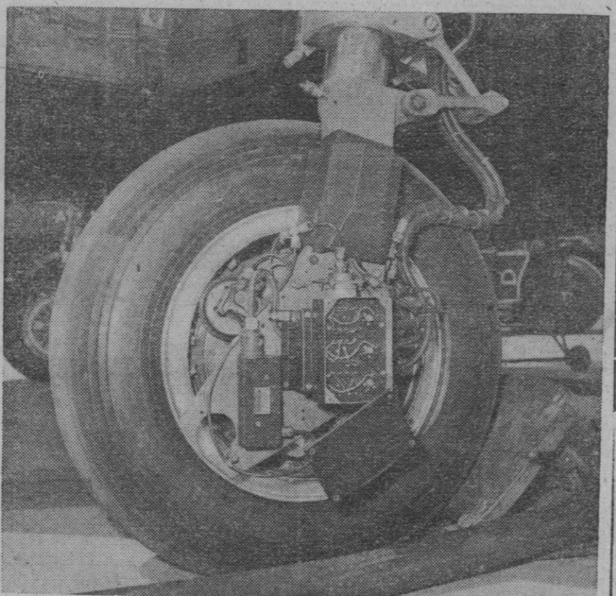
Las construcciones aeronáuticas no son una cosa simple. En realidad no hay casi nada sencillo en el mundo de hoy. Como demostración, puede valer el complicado mecanismo que ha sido inventado para dotar a los trenes de aterrizaje de los aviones de una mayor sensibilidad, procurándose así un aterrizaje más confortable. La foto nos lo muestra aplicado a un Vickers Supermarine Swift Mk. 7.
